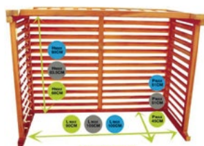
Modèle S Taille S 680x900x450mm (dim. intérieures) Modèle M Taille M 835x1050x510mm (dim. intérieures) Modèle L Taille L 950x1000x510mm (dim. intérieures)
