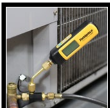
Vacuomètre MG44INT
