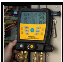
Manifolds numériques SM380VINT SM480VINT
