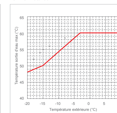
PUIZ-SW160/200YKA
