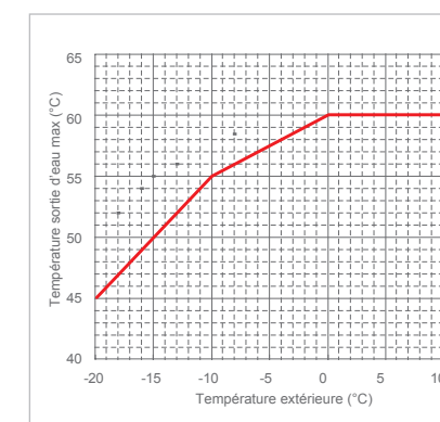
PUIZ-SW75VAA
